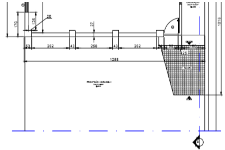
Planta Baixa - Ampliação Refeitório Escala 1/100
